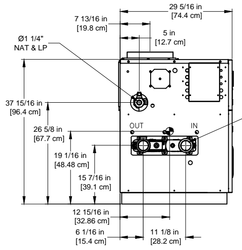
LEFT SIDE
